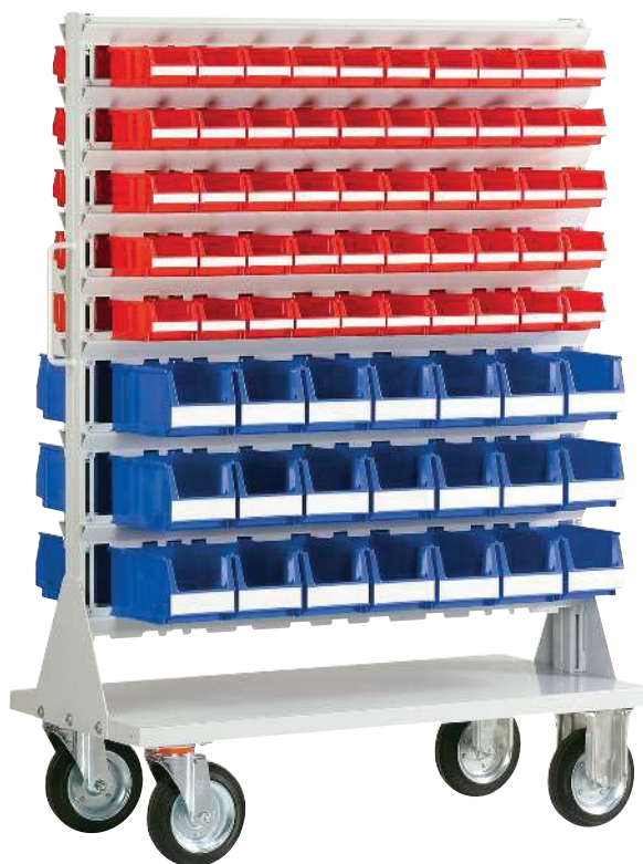
SB M 142 Einhängeregal BM 2seitig Aussenmasse: 1150x500x1570 mm mit 18 Aufhängeschienen
