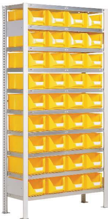
FA GR 3/36 Scaf. base SD fornito Misure esterne: 1000x300x2000 mm con 10 ripiani
